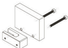
将贴尺工具安装在即将安装 AHBS 读数头的位置
